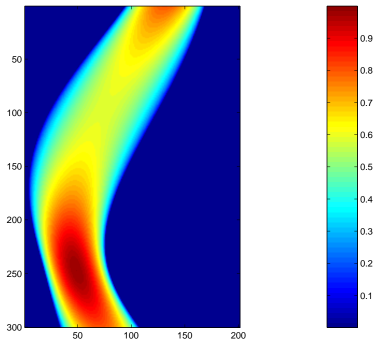
Radon-Transformierte der Ellipse ((s, \vartheta) \in [-1, 1] \times [0, \pi])
