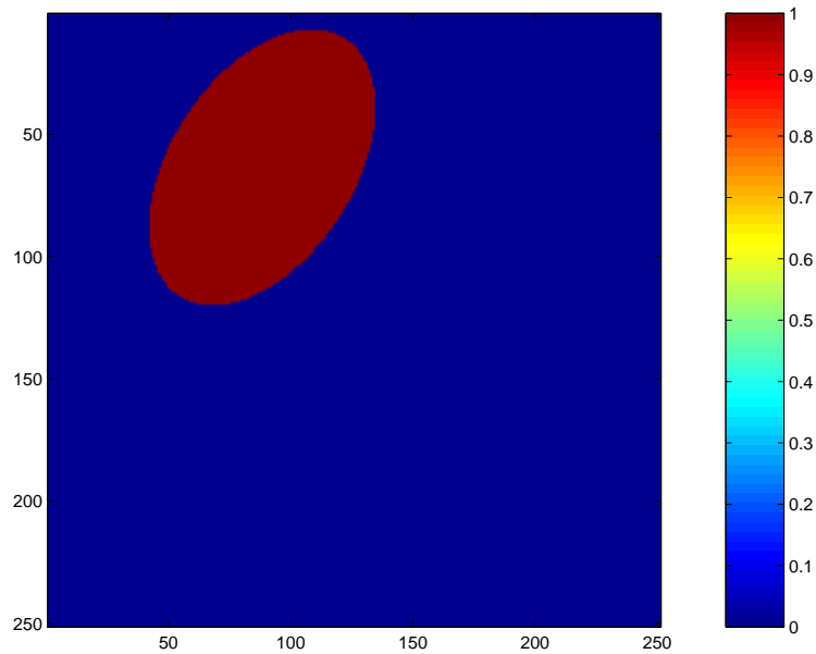
Charakteristische Funktion einer Ellipse
